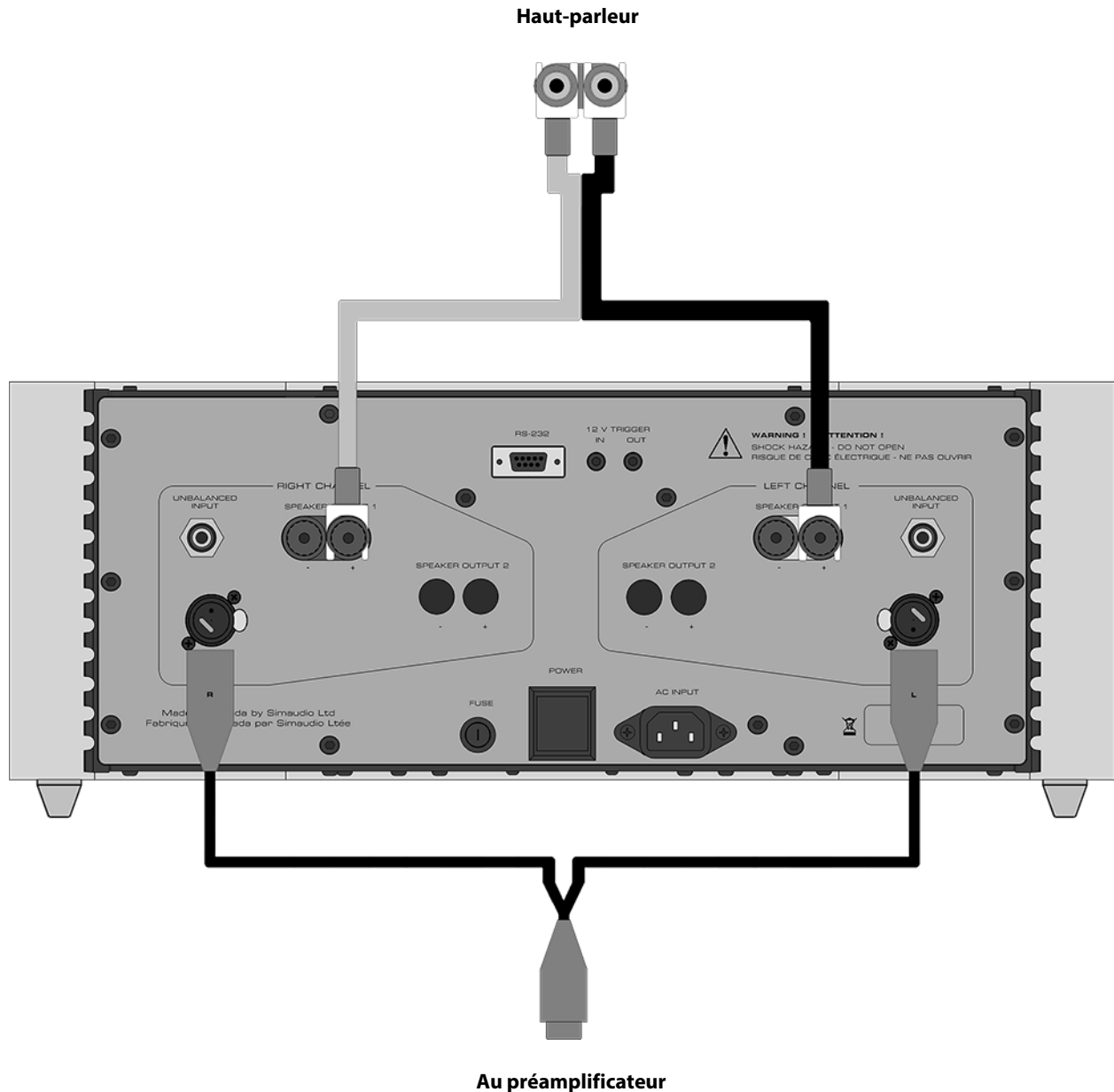
Figure 3: Utilisation en mode monaural du MOON 860A
