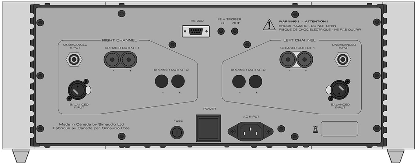
Figure 1: Panneau Arrière de l'amplificateur Moon 860A
