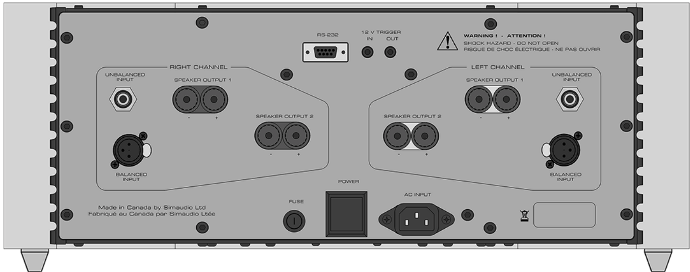
Figure 1: Panneau Arrière de l'amplificateur Moon 870A
