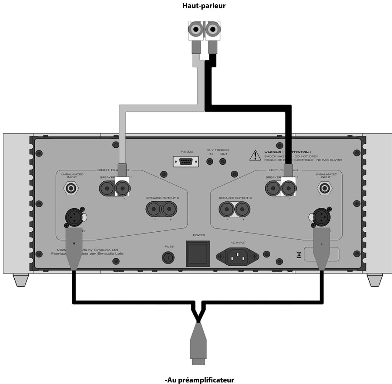
Figure 3: Utilisation en mode monaural du MOON 870A
