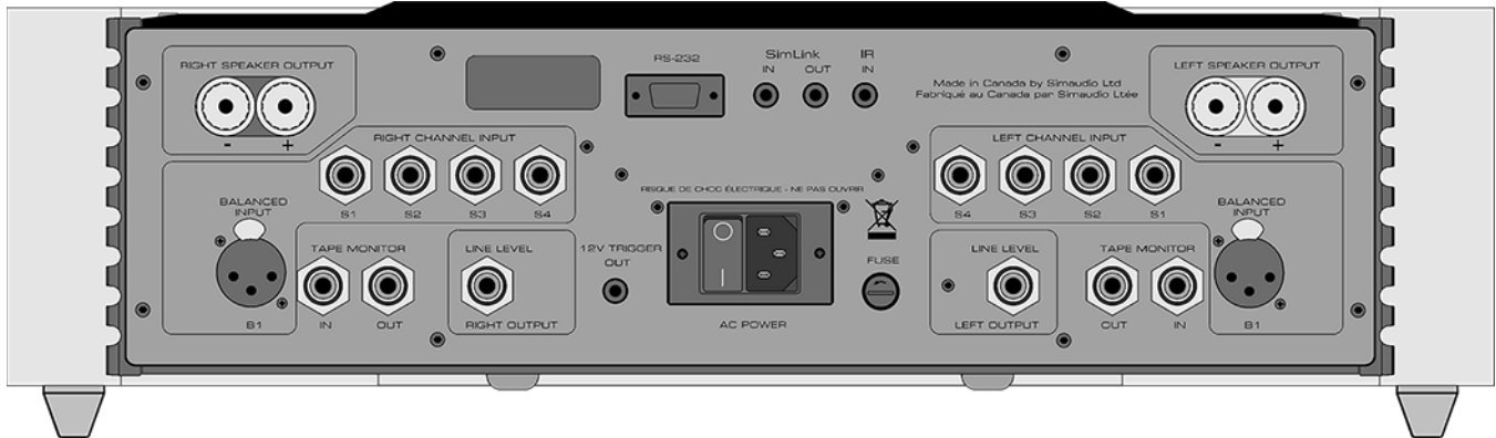
Figure 2: Panneau Arrière du 700i
